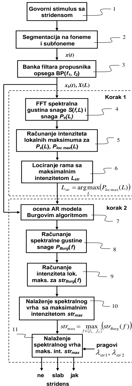
Slika 7.15 Algoritam detekcije stridensa pomoću FFT spektra i Burgovioog algoritma
