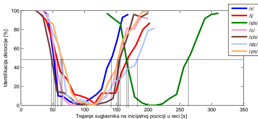
Slika 7.19. Identifikacione funkcije za glasove /c/, /č/, /dž/, /š/, /ž/, /r/, /l/.
