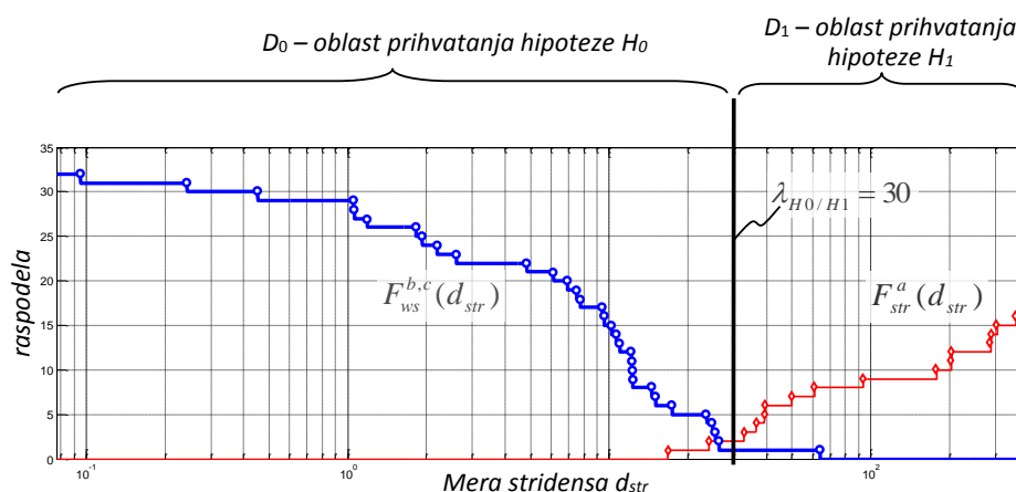
Slika 7.11 Testni slučaj 1. Distribucija mere stridensa: debela linija - F_{ws}^{b,c}(d_{str}) za subjekte sa korektnim izgovorom frikativa /š/ bez stridensa iz grupa (b) i (c), tanka linija - F_{str}^a(d_{str}) za subjekte sa stridensom – grupa (a). Prag odluke \lambda_{H0/H1}=30 dobijen je primenom kNN klasifikatora sa 3 najbliža suseda.
