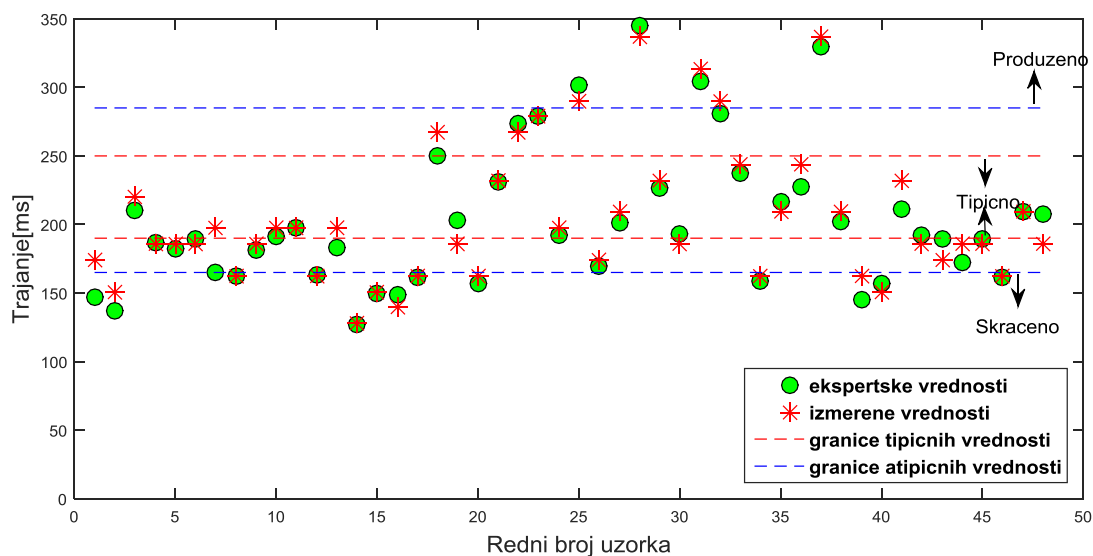
Slika 7.22. Trajanje glasa /š/ mereno na uzorcima iz baze patoloških govora - odrasli
