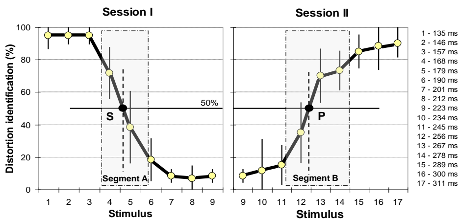
Slika 7.18 Identifikacione funkcije za glas /š/.
